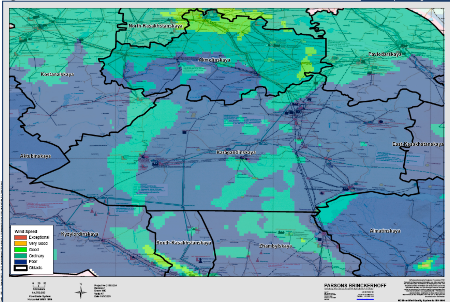
Рис.1 Карагандинская область. Карта с обозначением категорий скорости ветра на высоте 80 метров.
