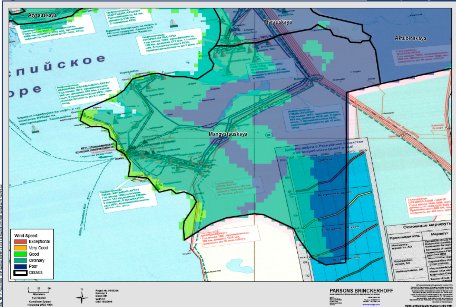
Рис.1 Мангыстауская область. Карта с обозначением категорий скорости ветра на высоте 80 метров.
