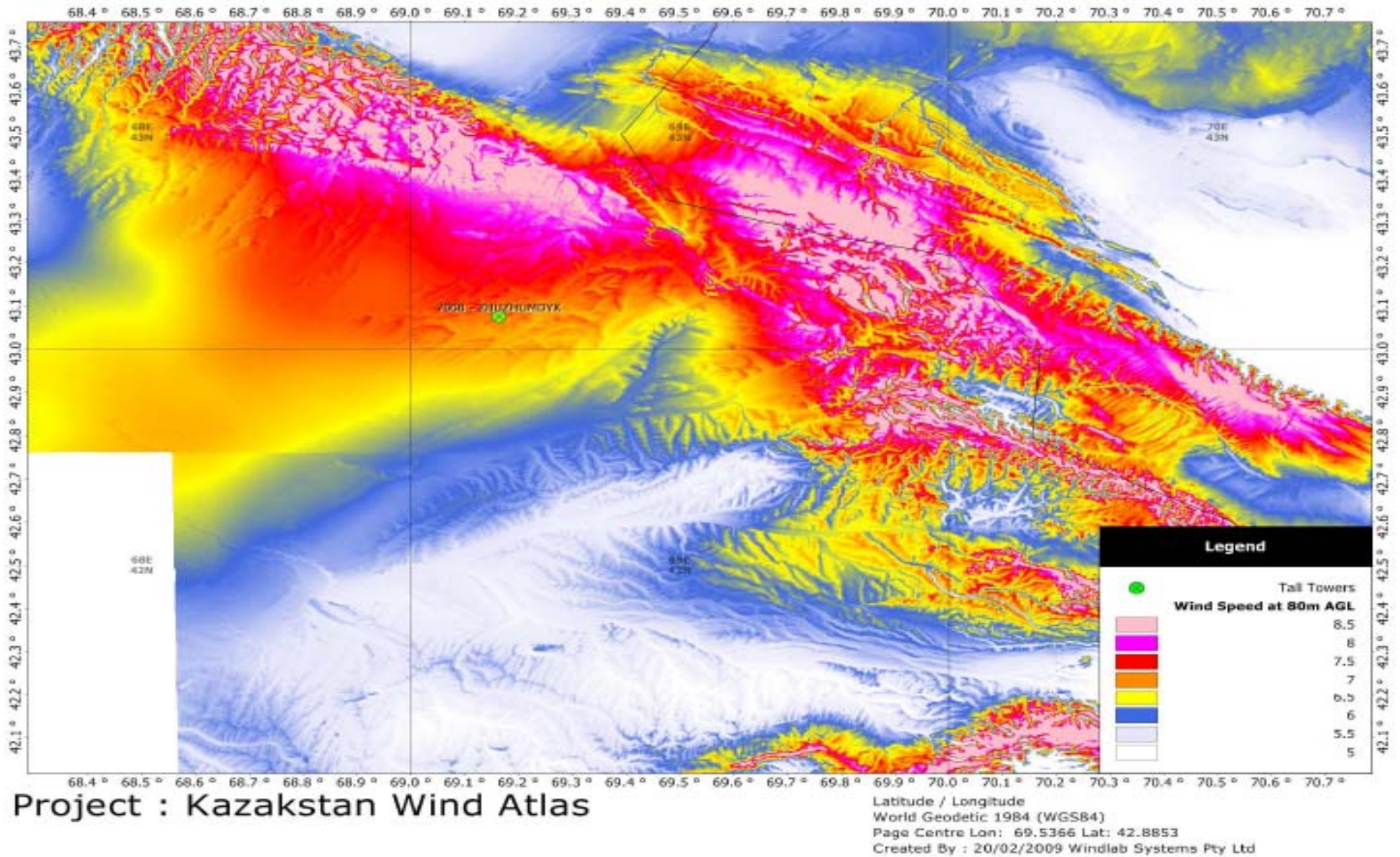
Рис. 2. Ветровая карта участка в районе пос. Жузумдык на высоте 80 м над уровнем земли и разрешением 100 м.
